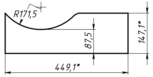
Поз.2 (Угольник) развертка
